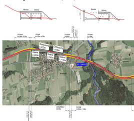
Optimierte Planungsvariante 2.3.1: Kombinierte Galerie- und Einhausungsvariante Frasdorf (940 m)
